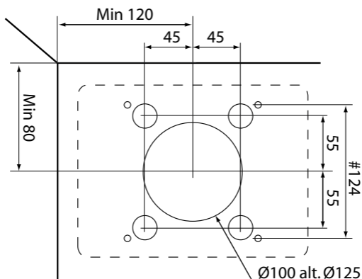
Pijpuitlaat voor verborgen installatie
